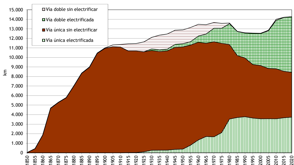
Evolution of the length of the network according to equipment (1850-2020) Evolución de la longitud de la red según equipamiento (1850-2020)
