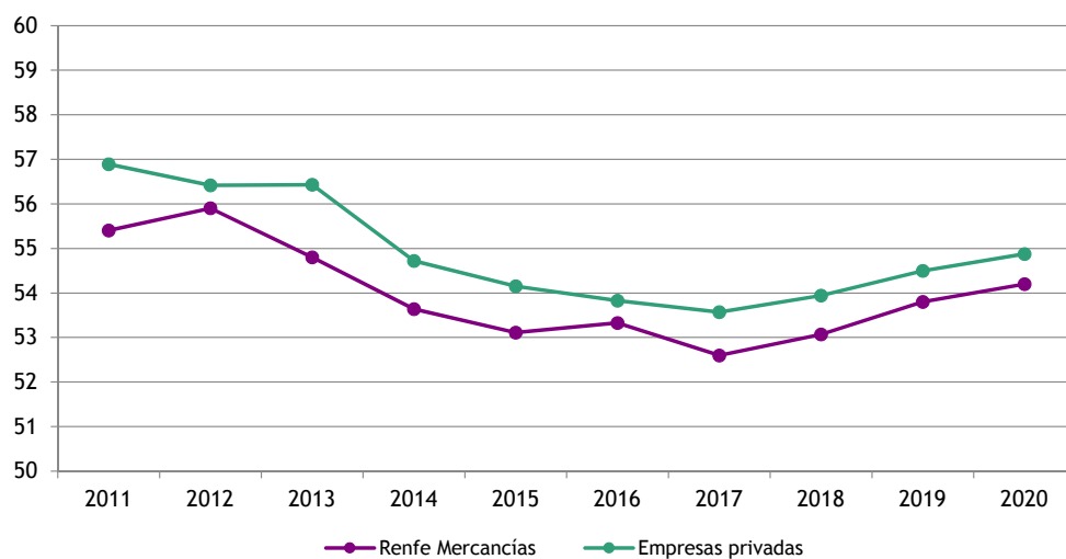
Velocidad media (km/hora) de los trenes de mercancías (2011-2020) Average speed (km/hour) of freight trains (2011-2020)
