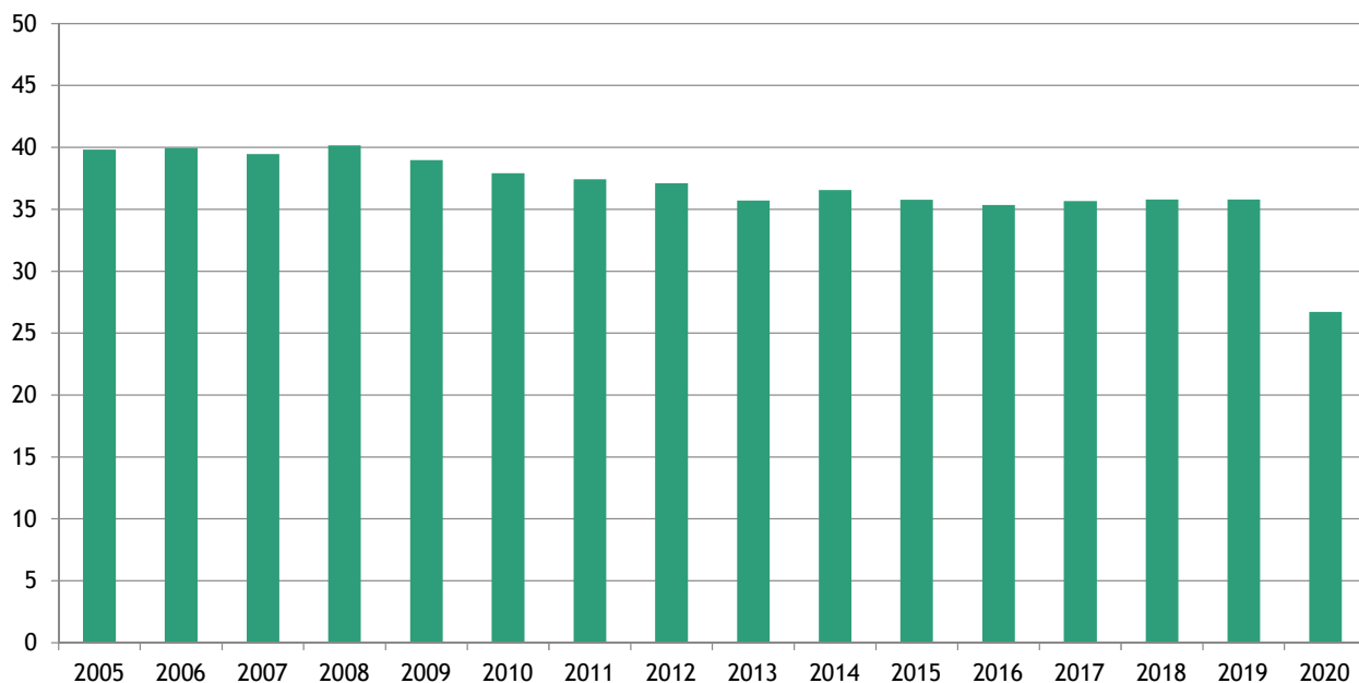
Densidad de circulación (Trenes.kilómetro/km de línea) (2005-2020) Traffic density (Trains.kilometre/km of line) (2005-2020)
