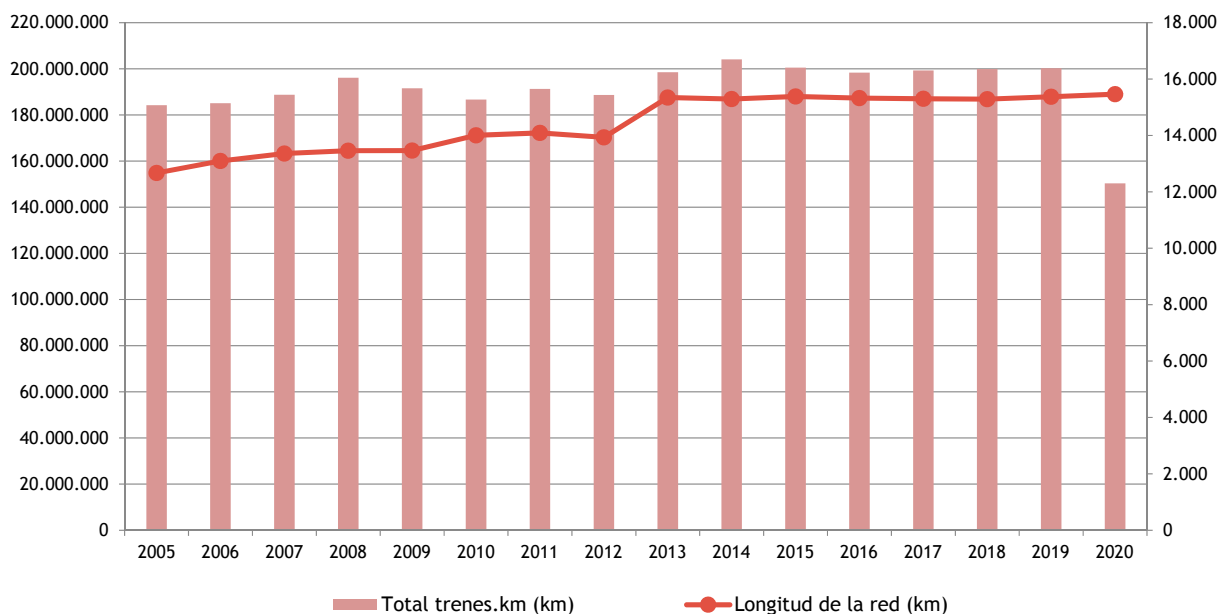
Recorrido anual en kilómetros de los trenes y longitud de la red (2005-2020) Annual run in kilometres of trains and length of the network (2005-2020)
