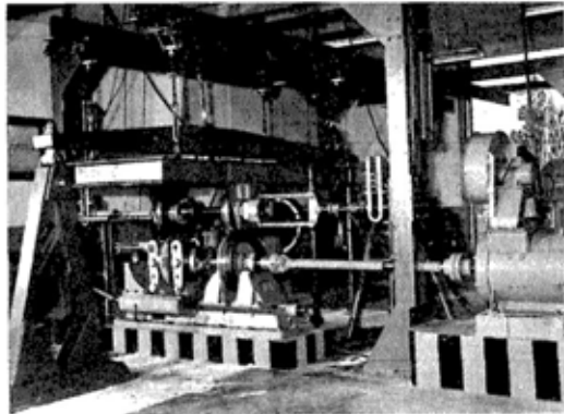
Banco de ensayos para eje a escala reducida (1:2,5).
