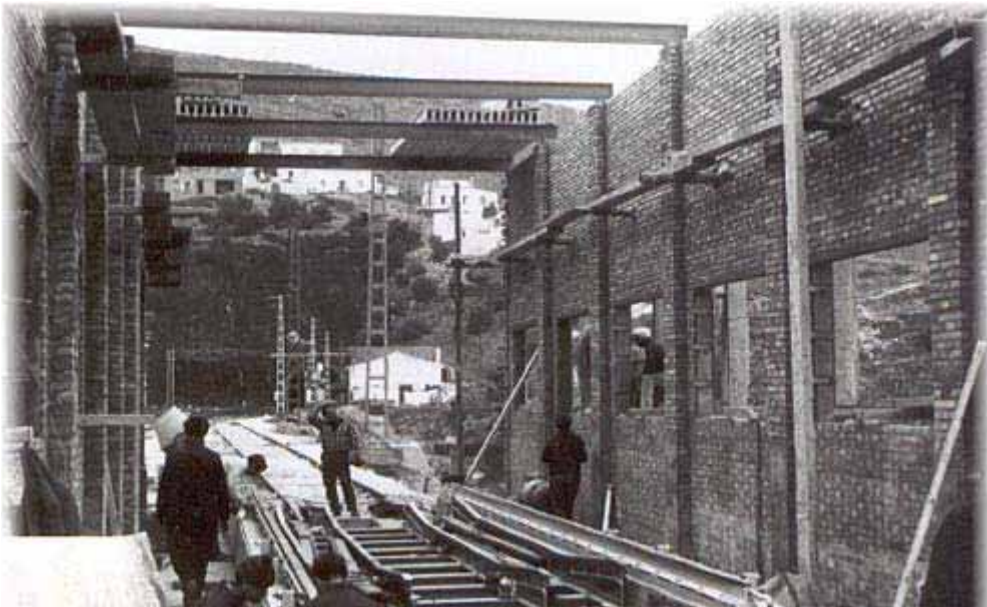
Construcción de del cambiador de Portbou en 1969 (Foto: Francisco Uriz)
