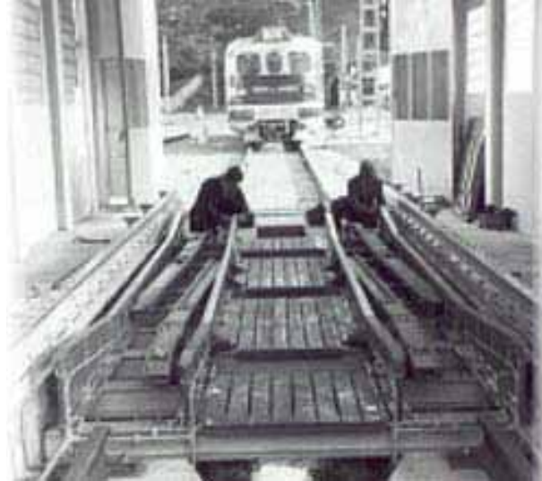
Cambiador de Portbou con máquina diésel 3000 al fondo (Foto: Francisco Uriz)
