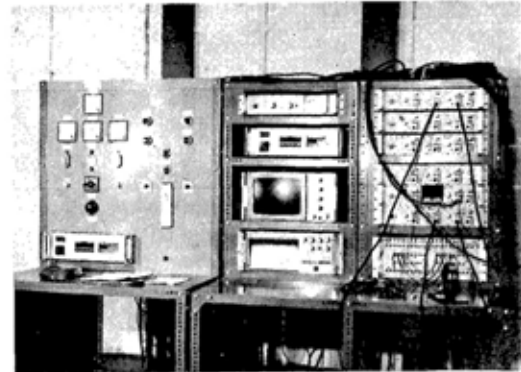
Pupitre de mados y aparatos de medida del banco de ensayos de ejes a escala reducida.
