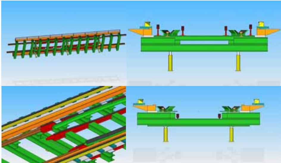
Cambiador único Talgo-CAF para trenes completos (TCRS 3). Fuente: TRIA
