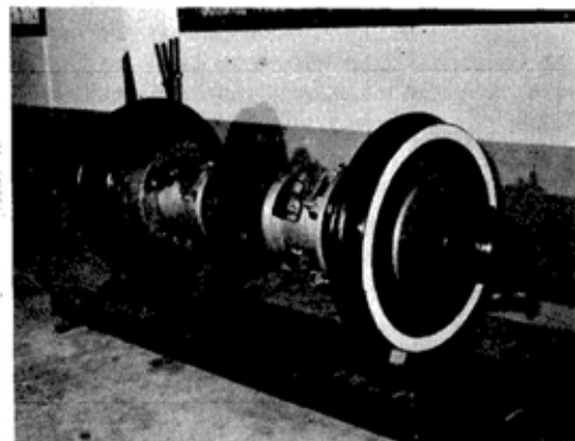
Ejes de cambio automático de ancho de vía O.G.I.
