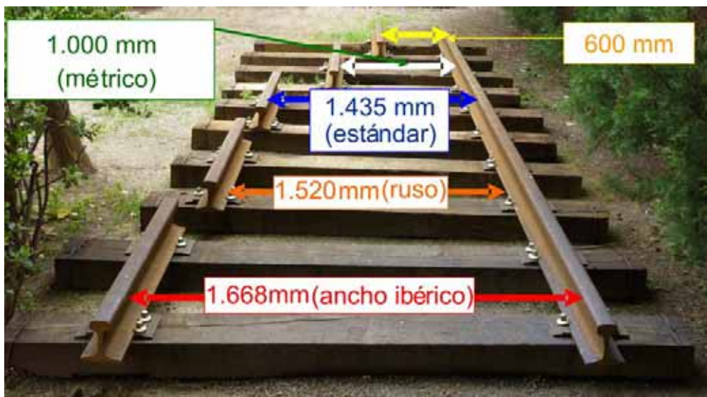
En el Museo del Ferrocarril de Vilanova i la Geltrú se muestra un montaje con diferentes anchuras de vía, desde el ibérico (1.668mm) hasta el de 600 mm
