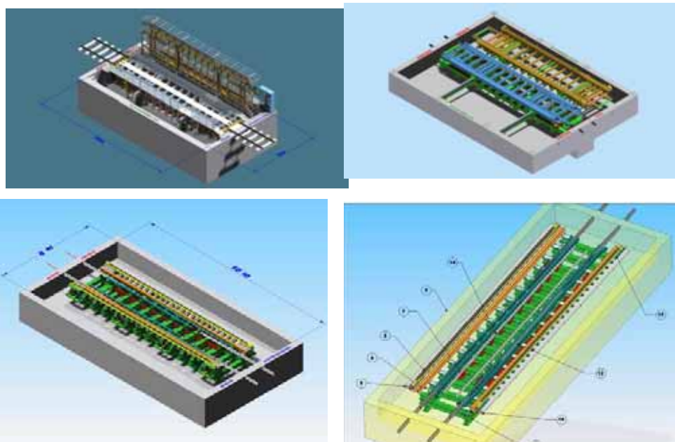
Esquemas de diversos cambiadores polivalentes: Arriba izquierda TCRS1 dual Talgo-CAF abatible; arriba derecha TCRS2 dual Talgo CAF horizontal; abajo izquierda TCRS3 dual Talgo CAF plataforma única; abajo derecha TCRS4 universal
