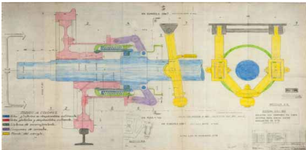
Plano del sistema O.G.I
