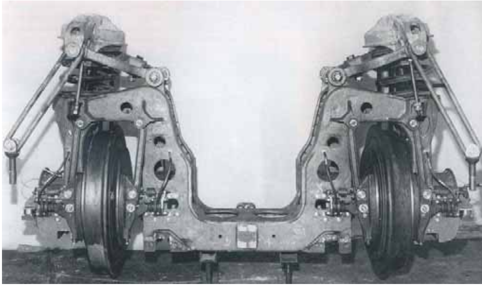
Rodal de ancho variable del Talgo III RD (1968). (Foto: Talgo)
