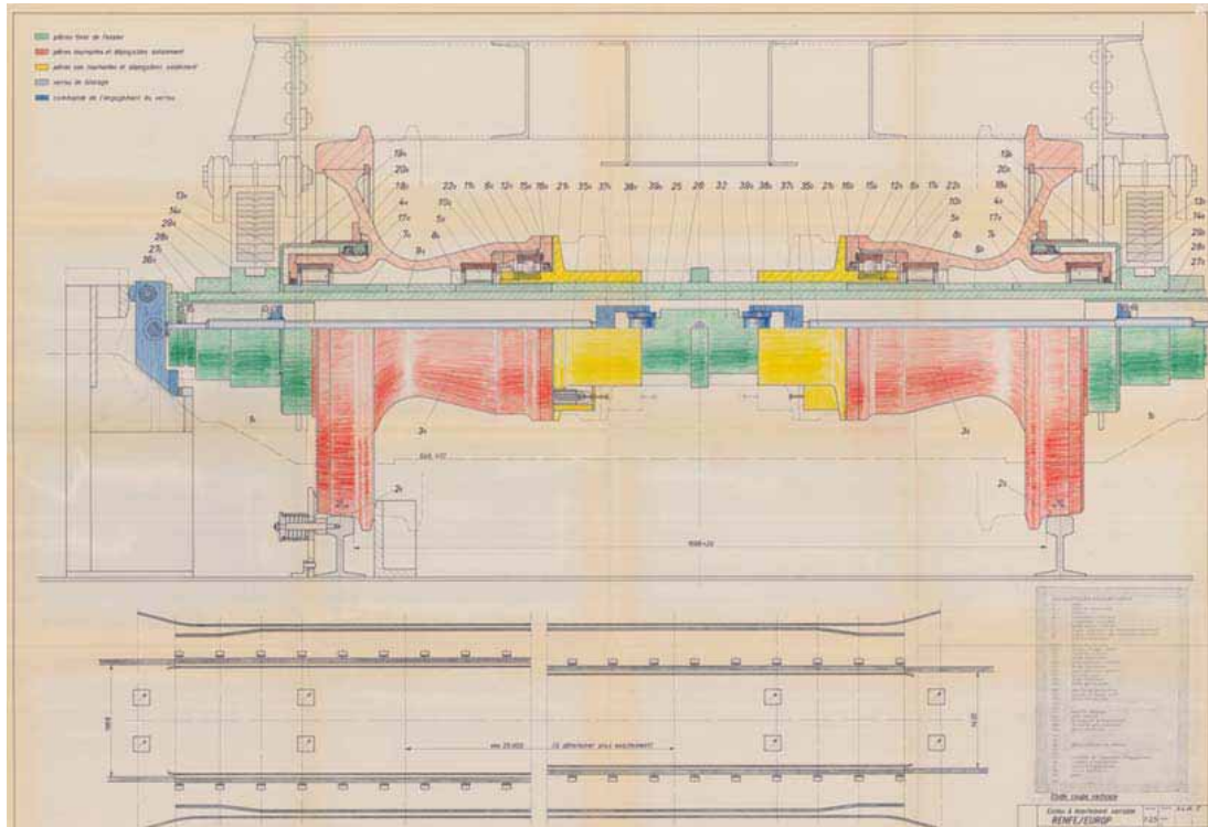
Plano del sistema Vevey
