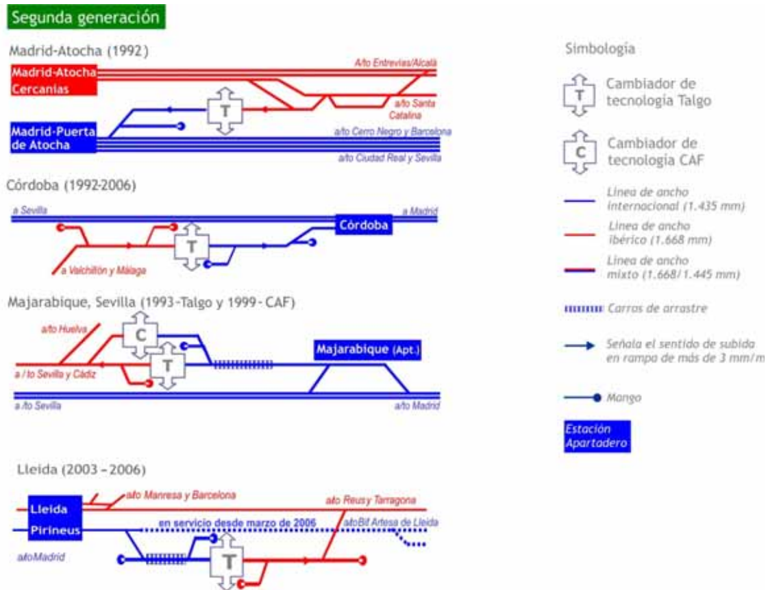
Esquema de los cambiadores de segunda generación
