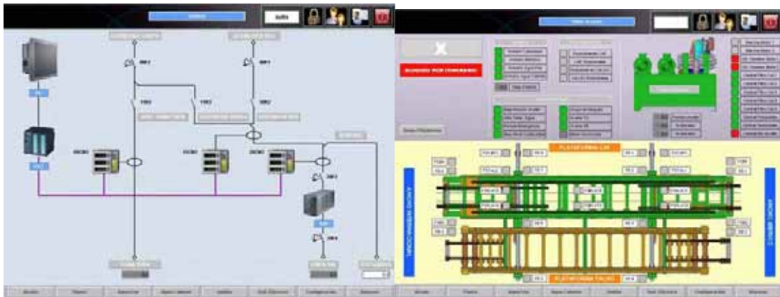
Pantallas de monitorización de los sistemas del cambiador
