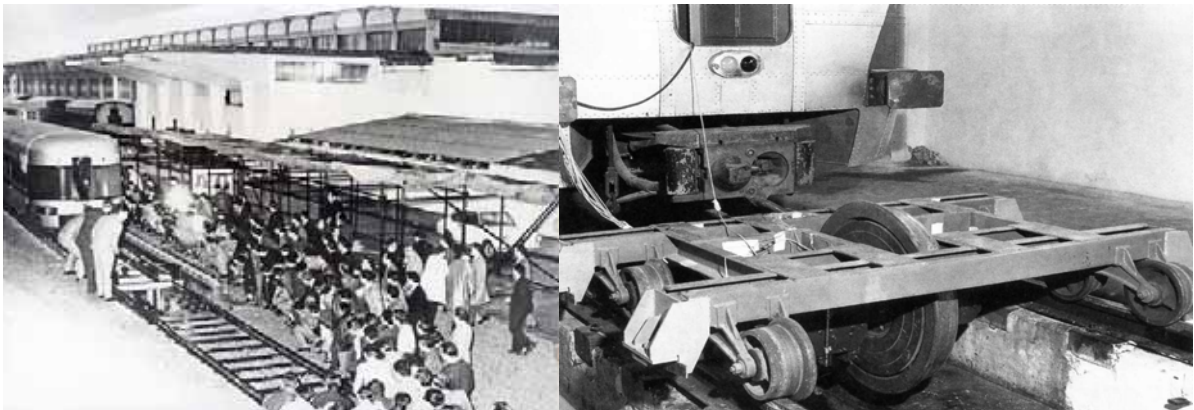
Primeras pruebas en Aravaca del sistema Talgo de rodadura desplazable en 1967 (RD). (Fotos Talgo)
