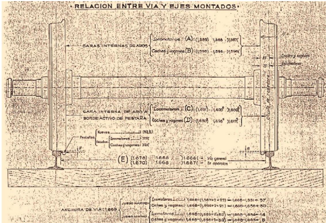
Relación entre ancho de vía y distancia entre ruedas. (Fuente: “Reducción del juego de vía” Departamento de Estudios y Reconstrucción de Renfe, de marzo de 1995)
